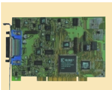
PH-220 – универсальный 4 или 8-канальный адаптер (с мезонином) канальный адаптер аналоговых телефонных, микрофонных и прочих линий связи
